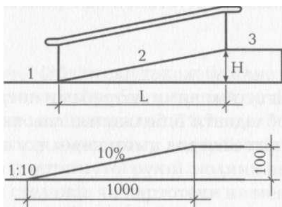
Рис.1. Строение пандуса.
